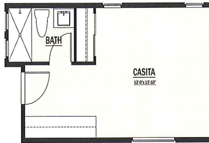
OPT. CASITA
